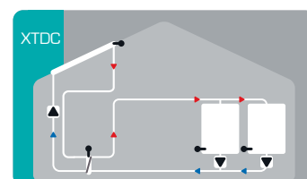
Solare con 2 accumuli, 2 pompe e scambiatore
