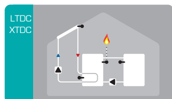
Solare con termostato e carico accumulo
