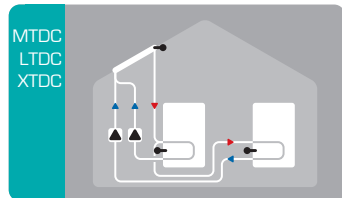
Solare con 2 accumuli e 2 pompe
