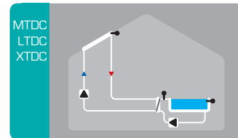
Solare con piscina e scambiatore
