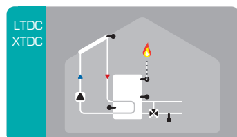
Solare con termostato e innalzamento ritorno
