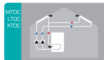
Solare con 2 collettori e 2 pompe
