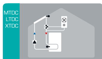
Solare con condizionamento 1 (collettore condiz.)
