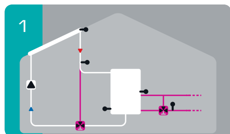
Solare con accumulo con funzione aggiuntiva Bypass solare e innalzamento ritorno
