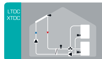
Solare con scambiatore, 2 accumuli
