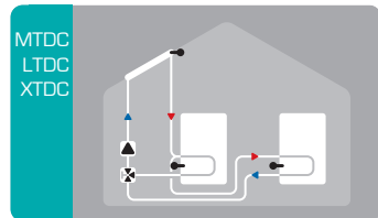
Solare con 2 accumuli e valvola
