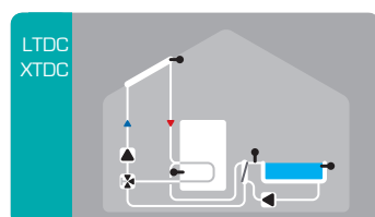
Solare con piscina, accumulo, scambiatore e valvola
