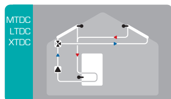
Solare con 2 collettori
