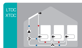
Solare con 3 accumuli e 2 valvole
