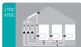
Solare con 3 accumuli e 3 pompe
