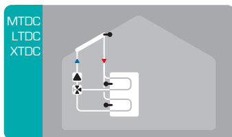
Solare con accumulo 2 zone
