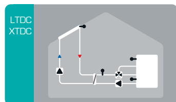
Solare con scambiatore e valvola di zona
