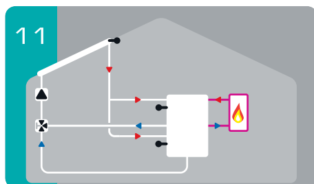
Solare con accumulo 2 zone e valvola deviatrice con funzione aggiuntiva termostato
