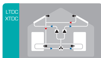
Solare con 2 collettori, 2 accumuli e 2 pompe
