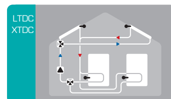
Solare con 2 collettori, 2 accumuli e 2 valvole
