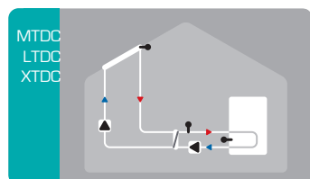
Solare con scambiatore
