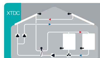
Solare con 2 collettori con 2 pompe, 2 accumuli, scambiatore e pompa
