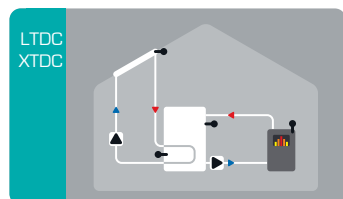
Solare con accumulo e caldaia a legna
