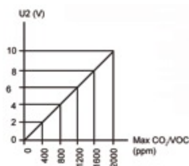
Diagramma funzionale CO 2 /VOC (Uscita U2)
