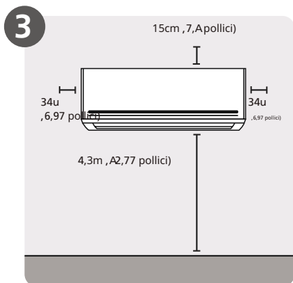
3 Seleziona la posizione di installazione
