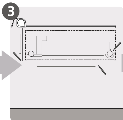
3 Determina la posizione del foro nella parete
