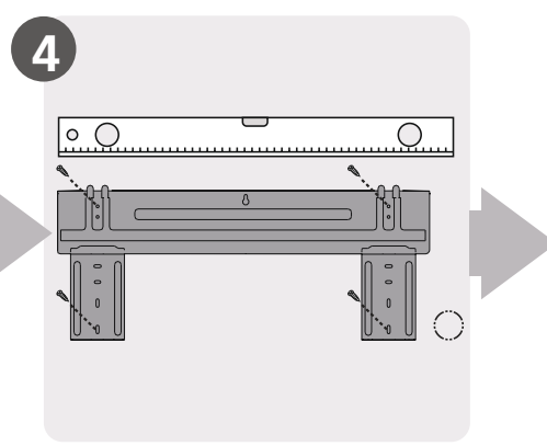
4 Fissa la piastra di montaggio
