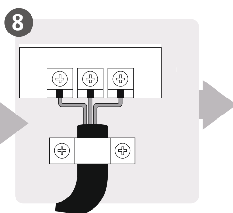
8 Collegare il cablaggio (non applicabile per alcune località in Nord America)
