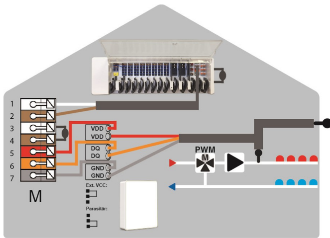
CAN bus dell'edificio e sensori ad 1-Wire
