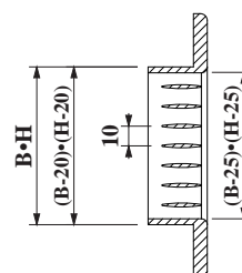
Sezione A-A
