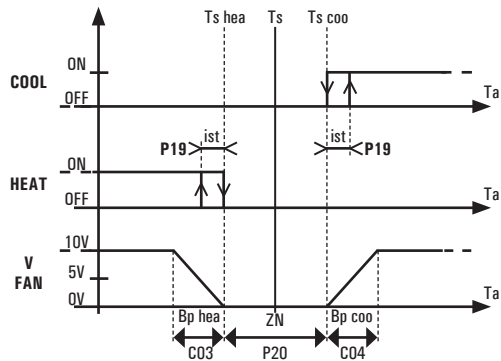
Fig. 15: Lo schema mostra il pilotaggio delle valvole in un impianto a 4 tubi con zona neutra. Analogamente, l'uscita valvola caldo (HEAT) di un sistema a 2 tubi verrà pilotata allo stesso modo, in questo caso la T_s (temperatura di setpoint) coinciderà con T_s ris in inverno e T_s raf in estate. Lo schema non tiene conto dell'eventuale azione del tempo integrativo e presuppone che l'uscita proporzionale del ventilatore (V FAN) sia configurata per azione diretta ( P05=0 ) e segnale 0..10V ( C15=0 ; C16=100 ). L'uscita proporzionale del ventilatore viene sempre spenta (0V) quando l'uscita della valvola, COOL o HEAT, è spenta (caso non visibile sullo schema).
