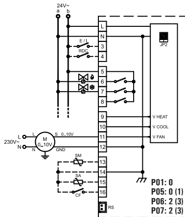
Fig. 9: Schema di collegamento per pilotaggio di due attuatori on/off a 24V ~ per impianto a 4 tubi e pilotaggio proporzionale del ventilatore. Wiring diagram for 2 on/off 24V ~ actuators in 4 pipes system and proportional fan drive.
