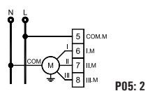
Fig. 13b. Collegamento di un ventilatore con motore a tre velocità. Connection of a fan with a three speeds motor.
